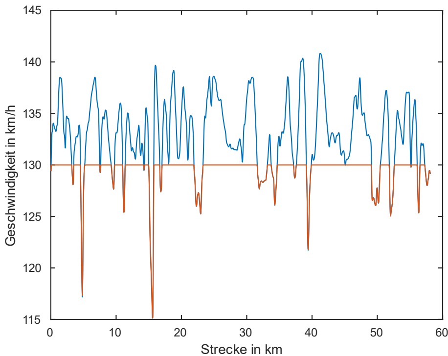
Abbildung 3-6: Beispiel der Anpassung eines Zeit-Geschwindigkeits-Profiles zur Verbrauchsimulation auf die zulässige Höchst- bzw. maximale Reisegeschwindigkeit von Reisemobilen und Caravans
