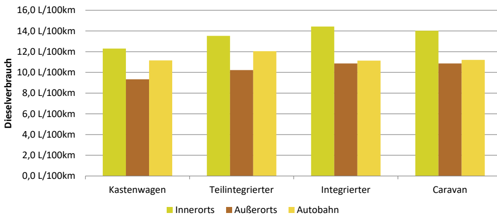
Abbildung 3-7: Treibstoffverbräuche [l/100 km] und THG-Emissionen [g CO 2 -Äquivalente je Fahrzeugkilometer] der Reisemobile für Innerorts-, Außerorts und Autobahnverkehr bei der jeweiligen Reisehöchstgeschwindigkeit.
