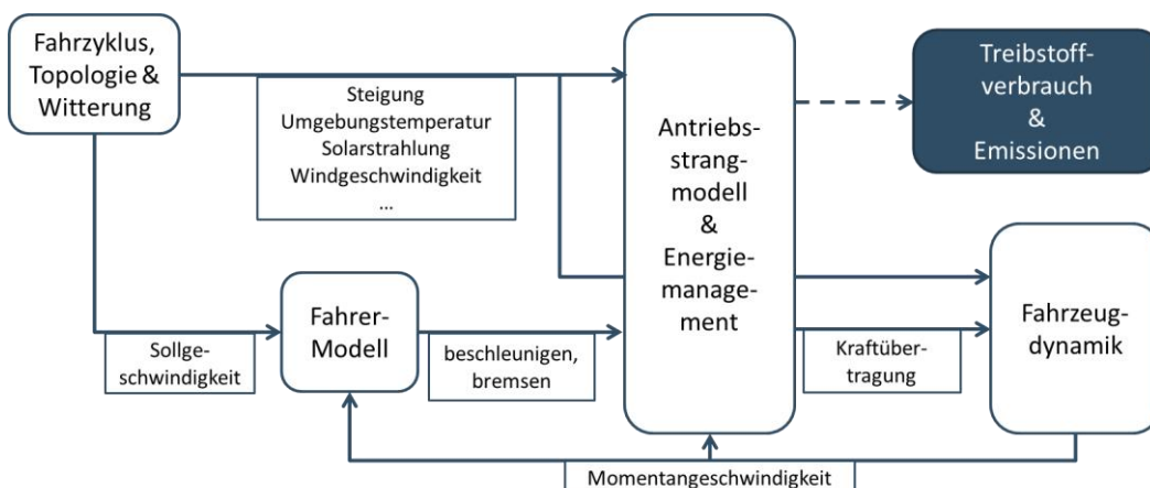
Abbildung 3-3: Schematischer Ablauf der längsdynamischen Fahrzeugsimulation in VEHMOD (eigene Darstellung)
