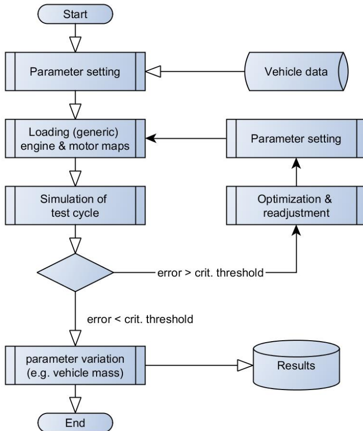
Abbildung 3-4: Vorgehen bei der Kalibrierung und Parameterjustierung der Reisemobile zur Verbrauchssimulation.
