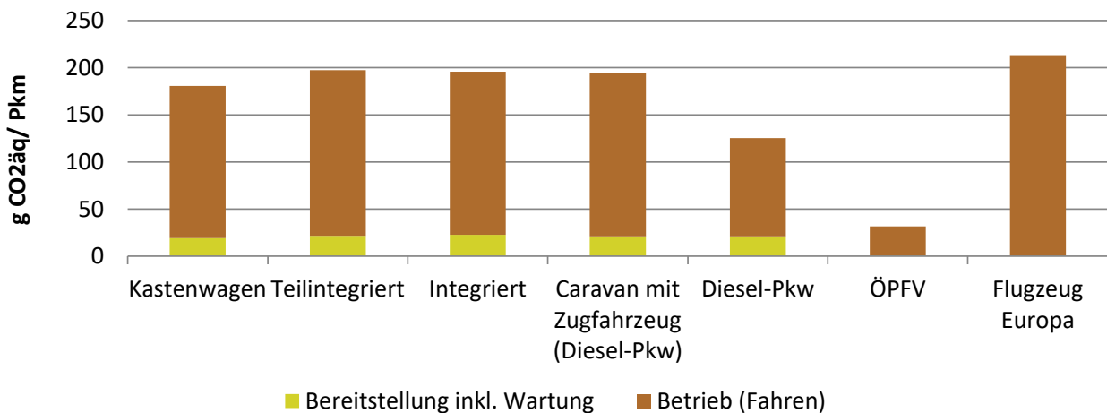
Abbildung 5-2: Vergleich Fernverkehrsmittel Emissionen je Personenkilometer bei einem Besetzungsgrad von 2 Personen für Reisemobile/ Caravan/ Pkw; Öffentlicher Personenfernverkehr (ÖPFV) und Flugzeug mit durchschnittlicher Besetzung
