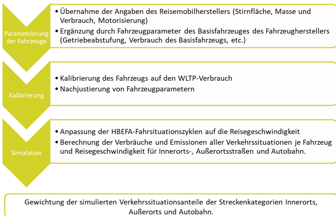
Abbildung 3-5: Vorgehen bei der Ermittlung der streckenspezifischen Verbräuche für Reisemobile für Innerorts-, Außerorts- und Autobahnstraßenabschnitte.
