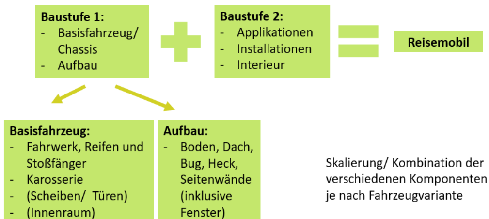
Abbildung 3-1: Aufbau des Modells zur Bilanzierung der Fahrzeugbereitstellung von Reisemobilen und Caravan
