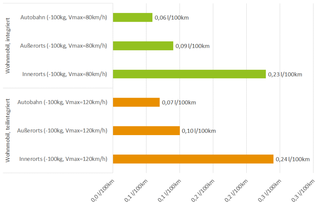
Abbildung 7-1: Kilometerspezifische Treibstoffersparnis bei 100 kg Gewichtsreduktion für Innerorts-, Außerorts- und Autobahnstraßenabschnitte. Eigene Berechnungen.
