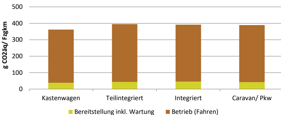
Abbildung 5-1: Durchschnittliche THG-Emissionen je Fahrzeugkilometer mit verschiedenen Reisemobiltypen und Caravans in Deutschland.
